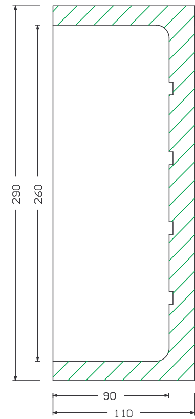
SEZ. A-A
