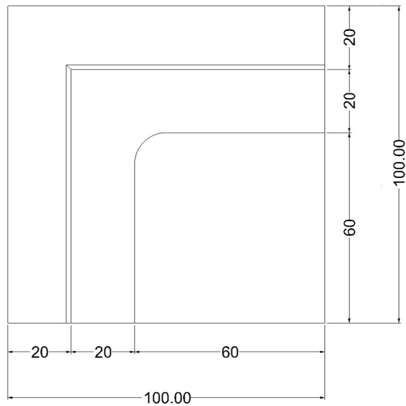
VISTA SUPERIORE
